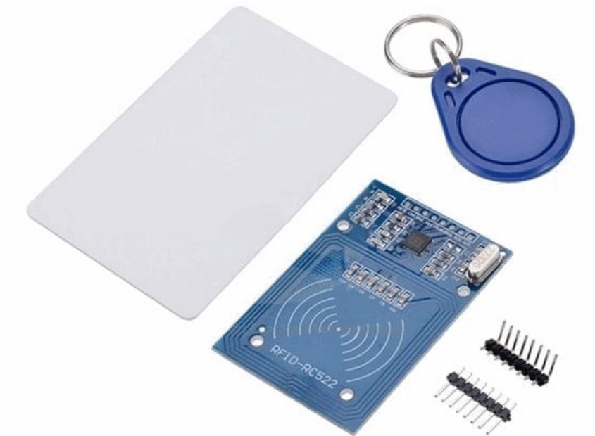
MFID-RC522 module
